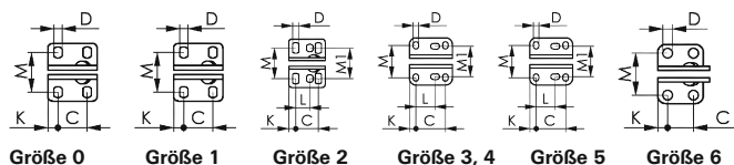
Maßtabelle
