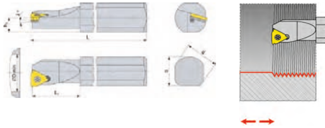
Abb.: Rechtsausführung Lieferung ohne Wendeschneidplatten.
