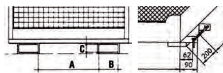
Einfahrtaschen-Innenmaße
