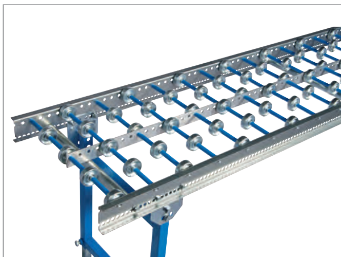
Typ AB148 mit Stahl-Röllchen
