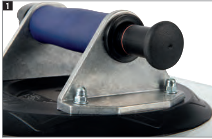
1 Aluminium-Körper mit eingebauter Handpumpe, besonders hohe Sicherheit durch visuelle Kontrolle des Vakuums am Pumpstößel. 210 mm Ø, Tragkraft ca. 120 kg.
