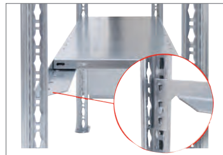
Mit Längenriegel
