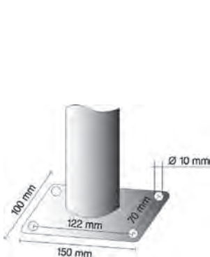
4 Dübelbefestigung
