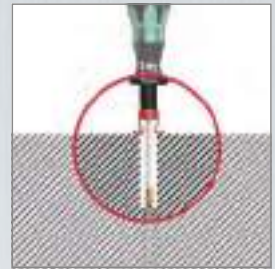
Bei tiefer liegenden Verschraubungen schiebt die Schraubkralle die Klinge hoch.
