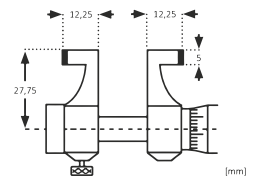
4305 0050-0100 [mm]
