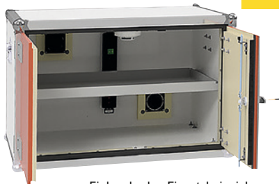
Einlegeboden Einsatzbeispiel
