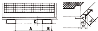
Einfahrtaschen-Innenmaße
