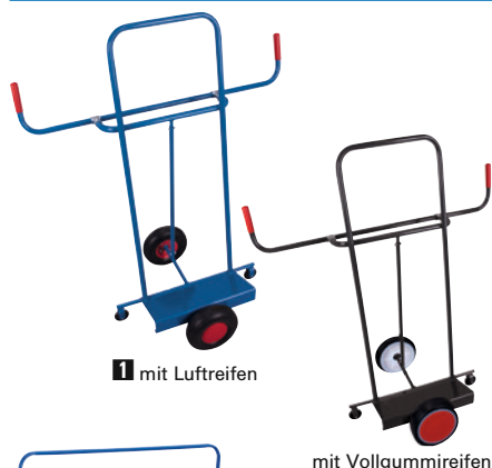
mit Vollgummireifen
