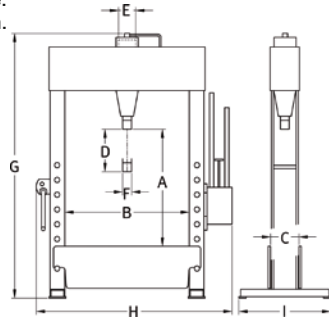
Pressplatte
