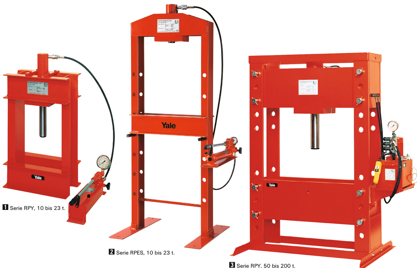
3 Serie RPY, 50 bis 200 t.
