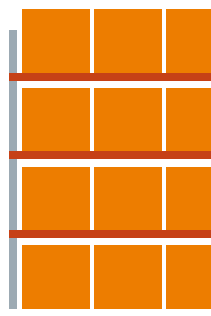
Grundfeld 1 Feld je 2700 mm 12 Palettenplätze
