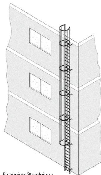
Einzügige Steigleitern.
