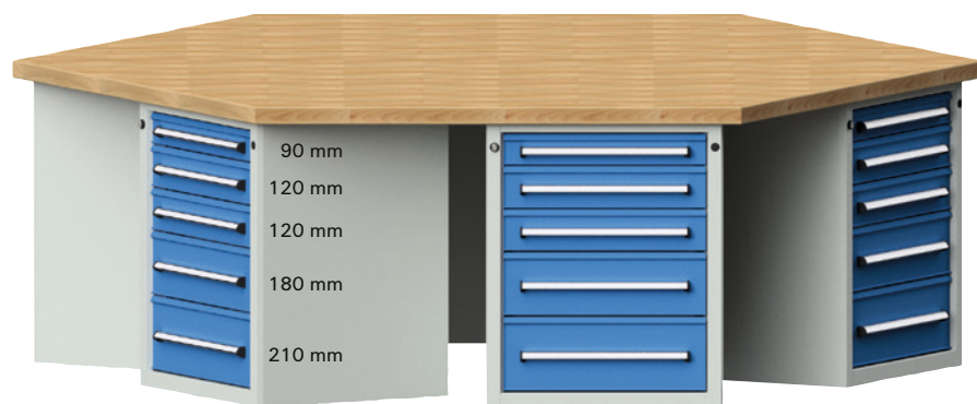
Platte Buche massiv, längsseitig riegelartig zahnverleimt, 50 mm stark.
